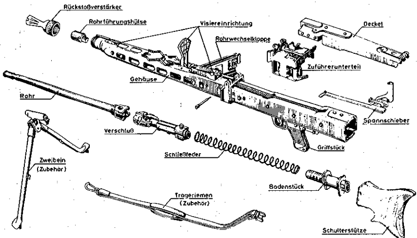
Baugruppenübersicht
