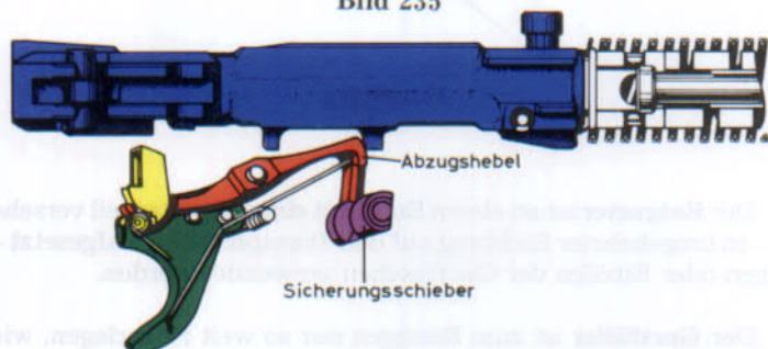
Abzugshebel hält Verschuß in hinterer Stellung
