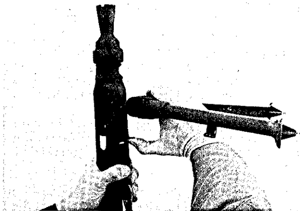
Zweibein abnehmen
