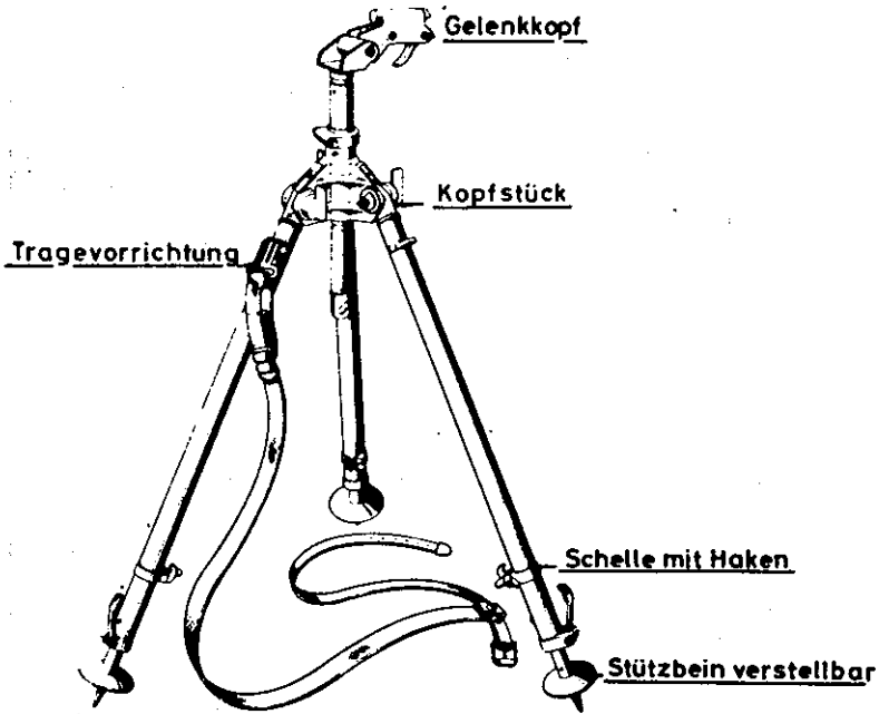
Fliegerdreibein
