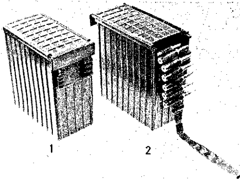
Patronenkasten DM40004 1 Deckel von rechts aufgeschoben 2 Deckel von links aufgeschoben
