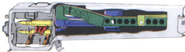
Patronentransport beim Rücklauf
