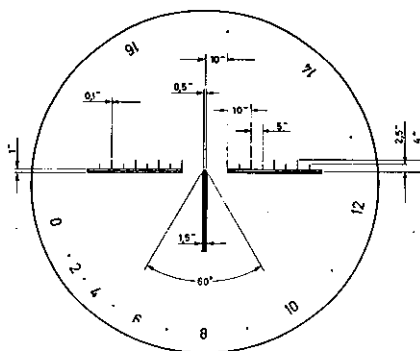
Zeichnungsmaße zum Strichbild
