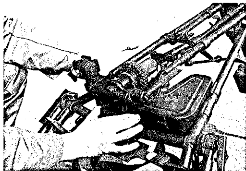
Oberlafette lösen
