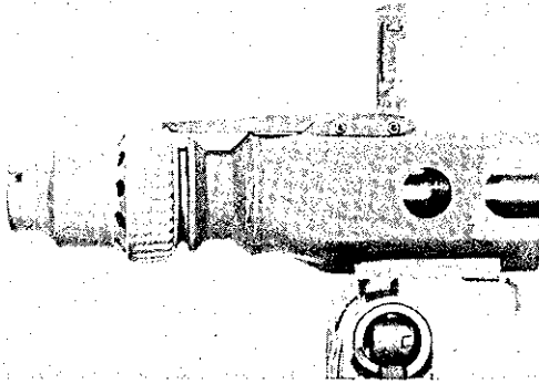
Aufgeschraubtes Manöverpatronengerät
