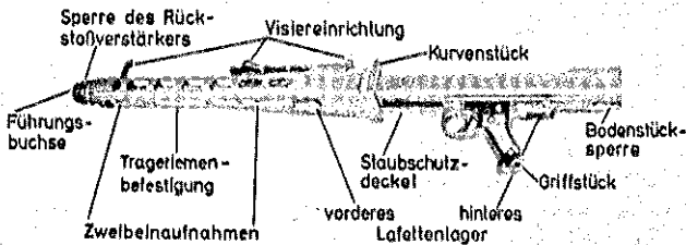
Gehäuse
