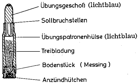
Aufbau einer Übungspatrone 7,62 mm \times 51 DM18
