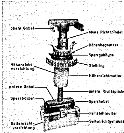
Richtvorrichtung
