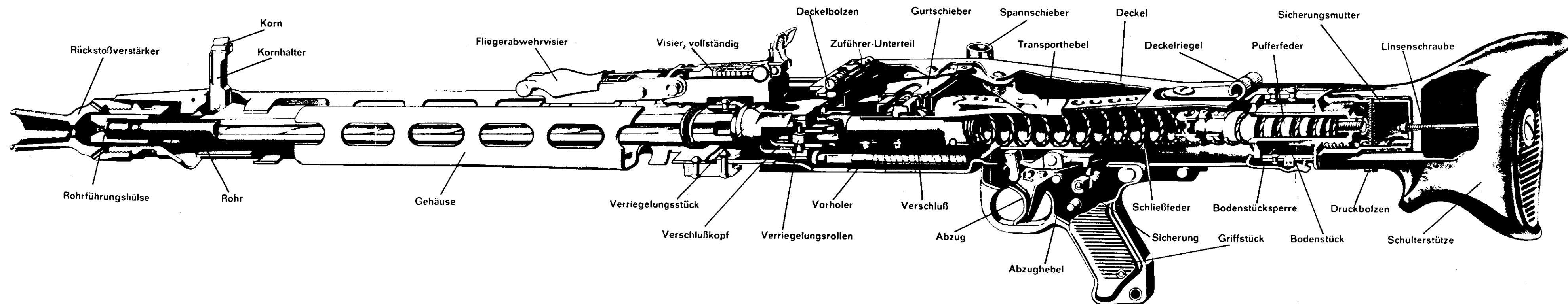
Schnittbild
