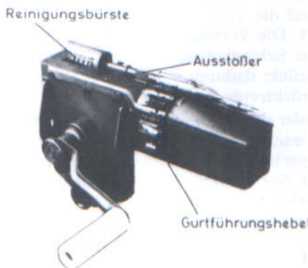
Entgurten
