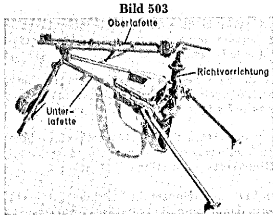
Feldlafette-MG
