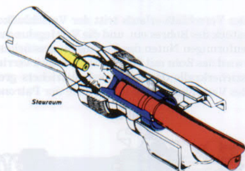
Rückstoßverstärkung
