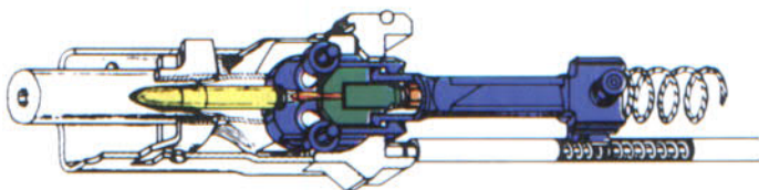
Rohr mit Verschuß verriegelt
