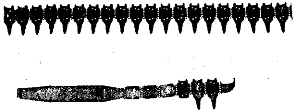
Teilansicht des Patronengurts DM1 und Einführstück (leer von unten gesehen)
